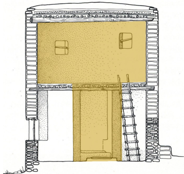
Abb. 10: Schnittzeichnung zur Rekonstruktion neolithischer Rundbauten auf Zypern mit einer von zwei zentralen Pfeilern getragenen Zwischenebene (KALAVASOS-TENTA, S. 40)
